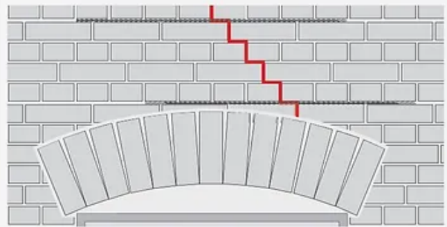
Risse im Bereich von Stützen/Bogenstützen Cracks in the area of lintels and arches
