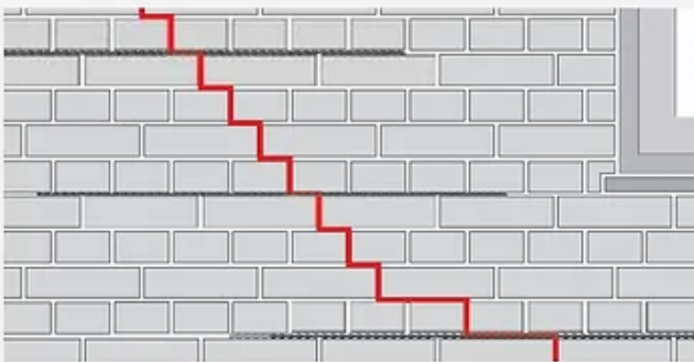
Risse im Bereich von Öffnungen Cracks in the area of openings
