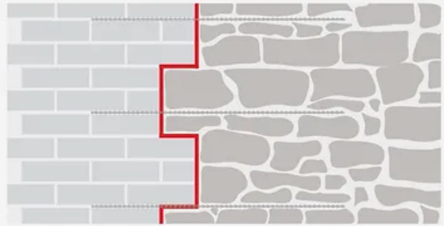
Risse im Mauerwerk Anchoring e. g. of natural stone facing
